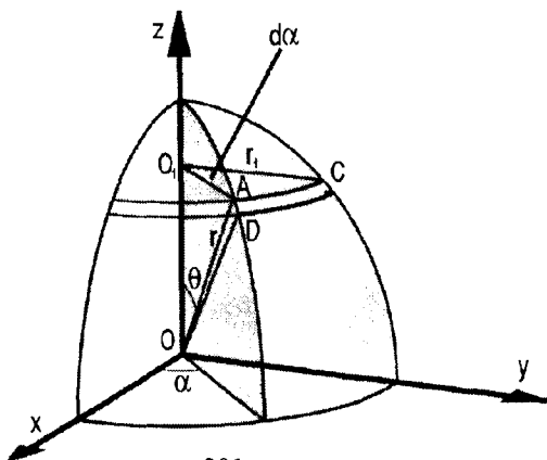
201-a rasm. Elektromagnit to‘lqinlar energiyasini aniqlashga doir.
