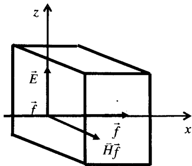
201-rasm. Elektromagnit to'lqinlarning paydo bo'lishi
