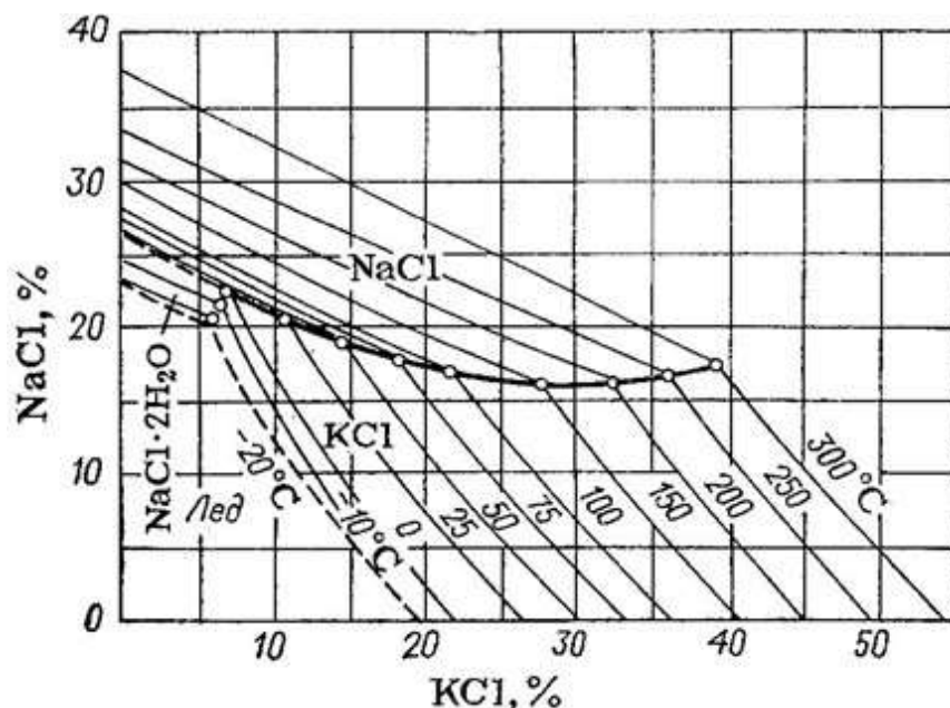
Политермическая диаграмма растворимости в системе KCl-NaCl-H 2 O (масс. %).
